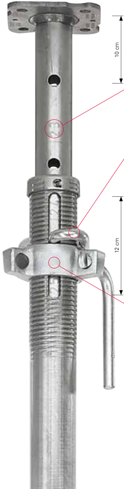
Pituusmerkintä PEP Ergo -holvitukissa on selvästi näkyvillä.
